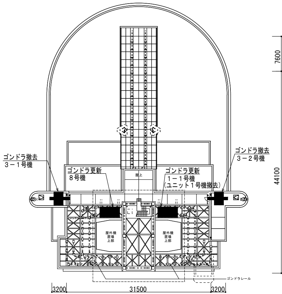
PH3階平面図 1/500
