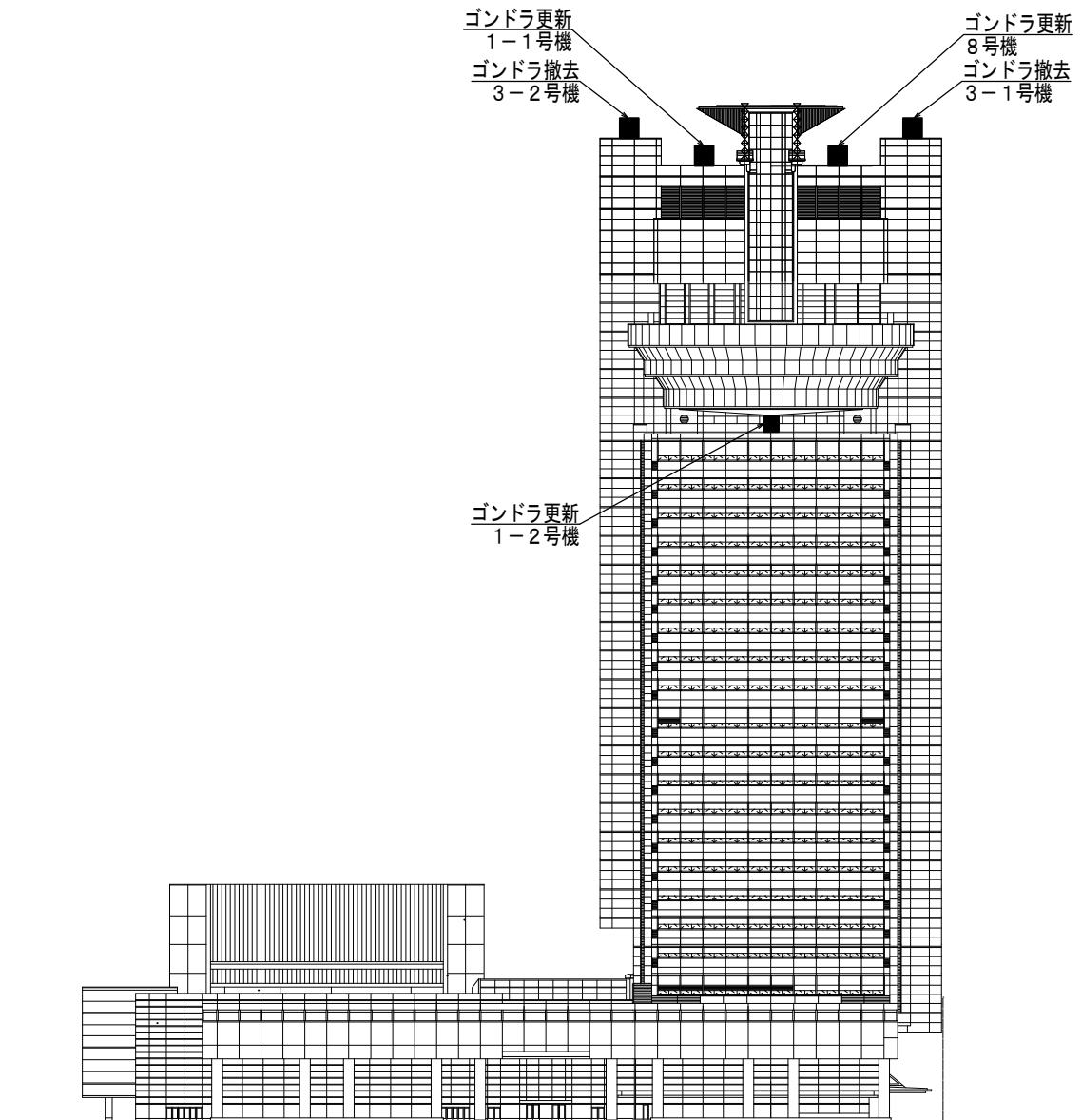
北側立面図 1/500
