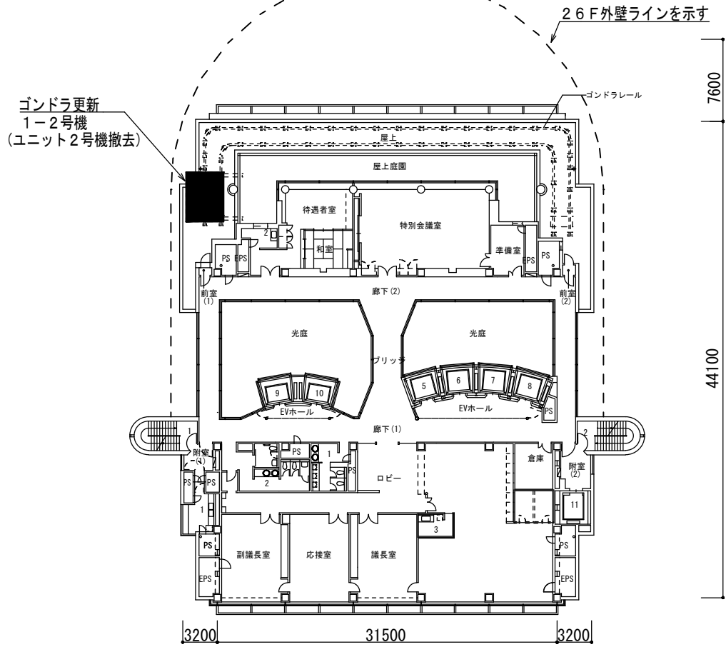
23階平面図 1/500
