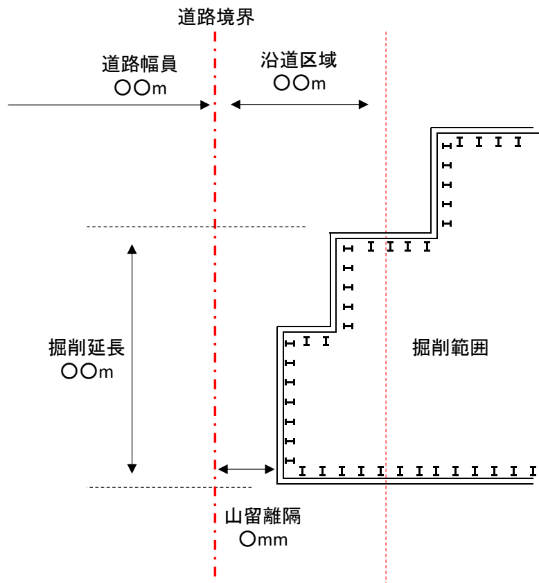
平面図
