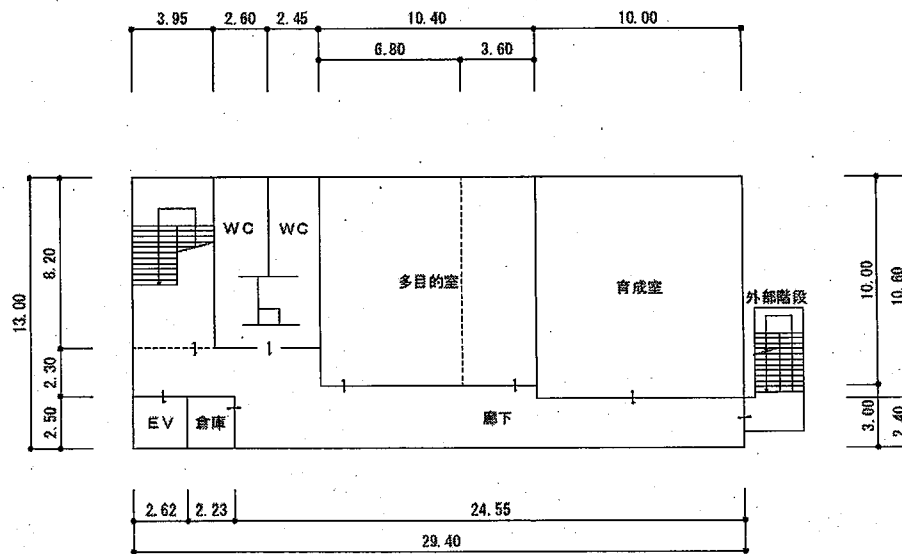
3階平面図
