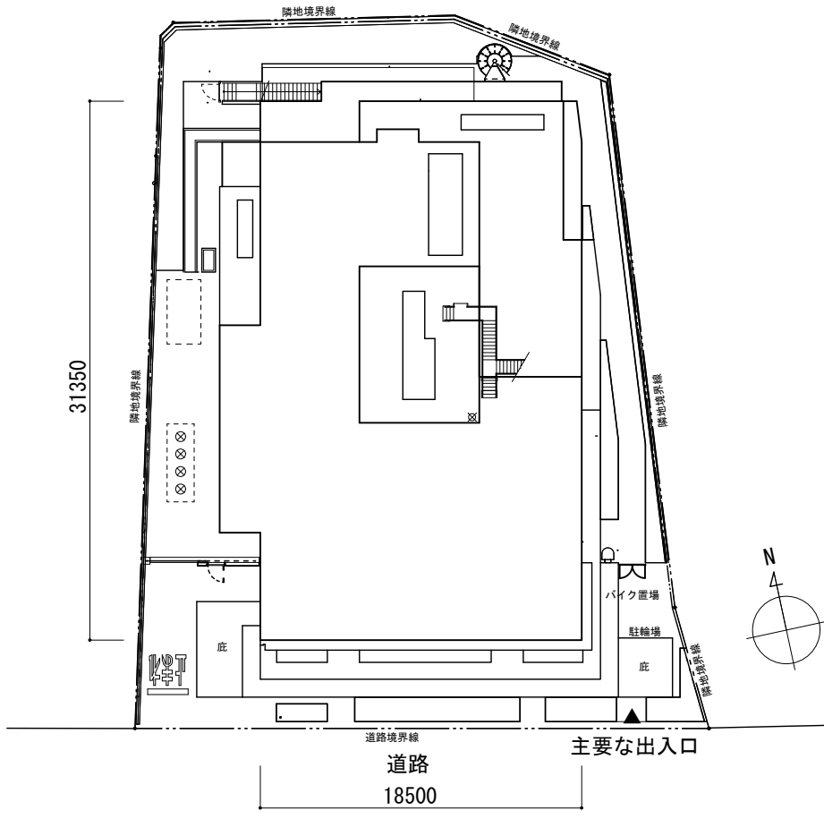
配置図 S=1/400
