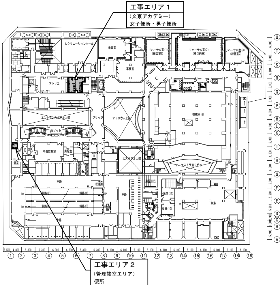
地下1階平面図 S=1/1000
