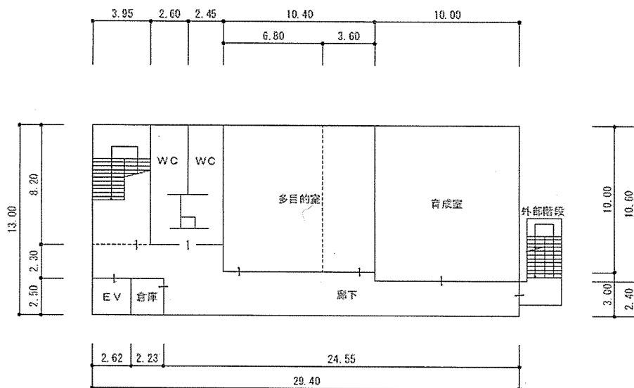
3階平面圖
