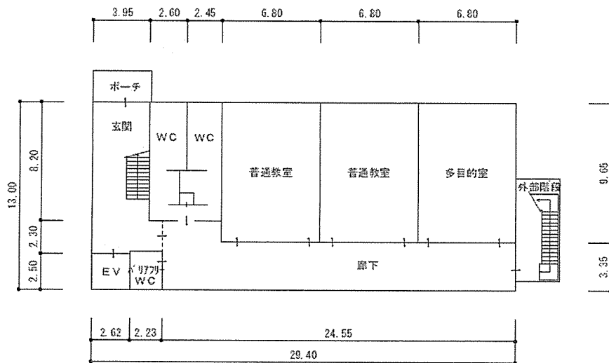
1階平面圖
