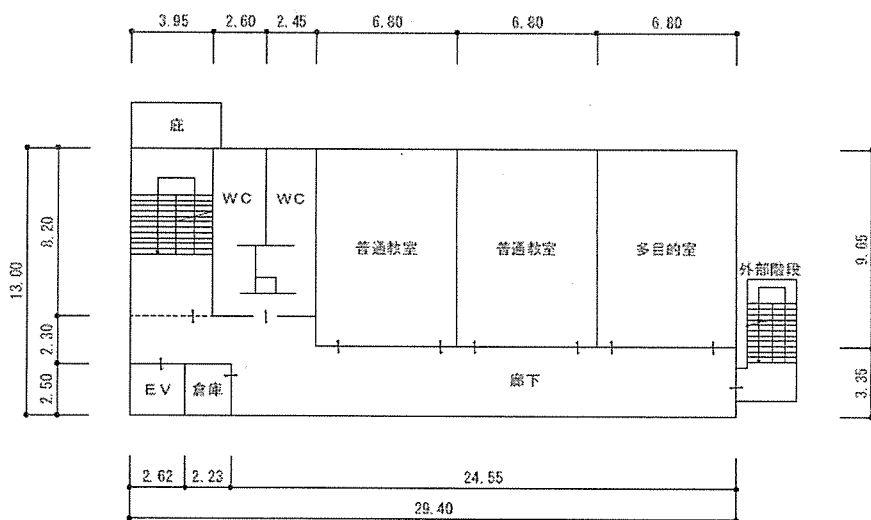
2階平面圖
