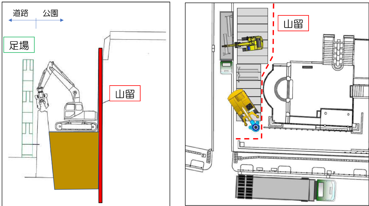
西側擁壁の作業イメージ図
