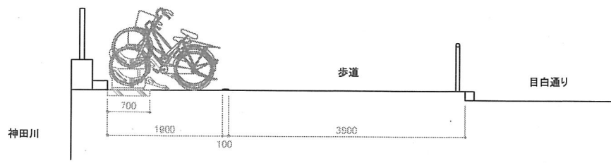
A-A'断面図
