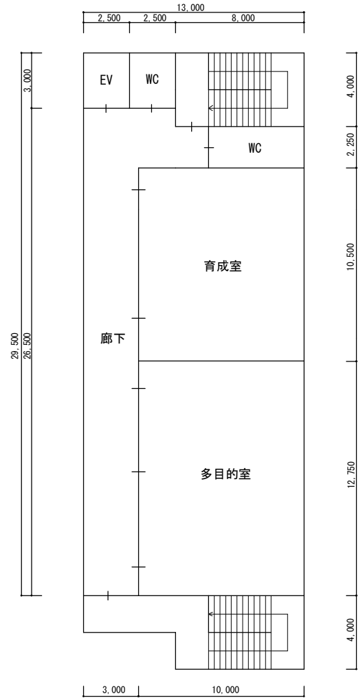
3階平面図
