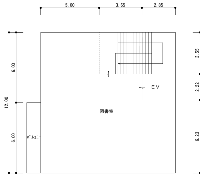
1階平面図
