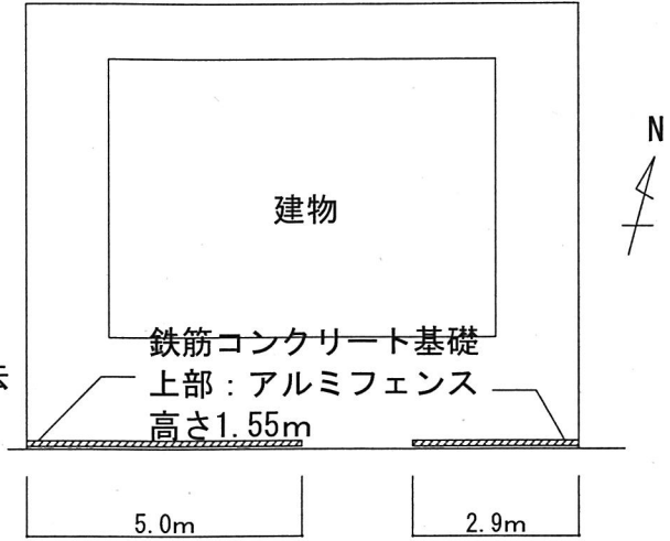
改修設計平面図 1/100
