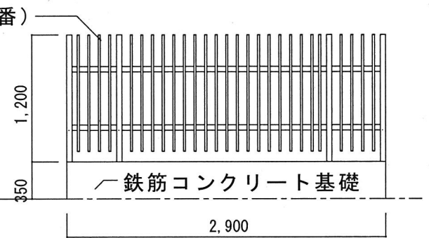
改修設計立面図 (東側) 1/100
