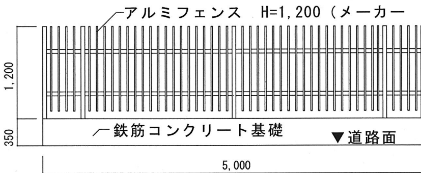
改修設計立面図 (西側) 1/100
