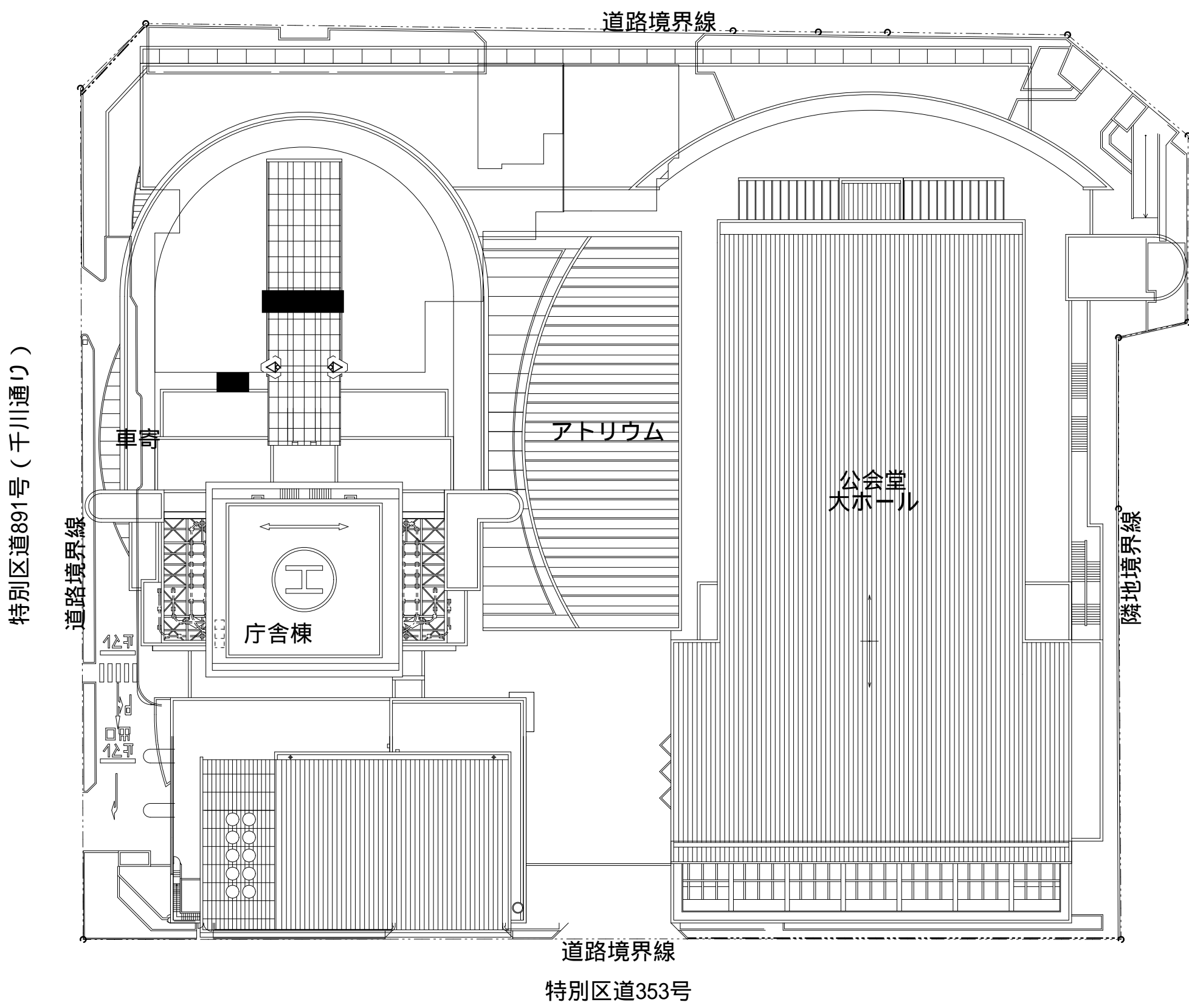
配置図
