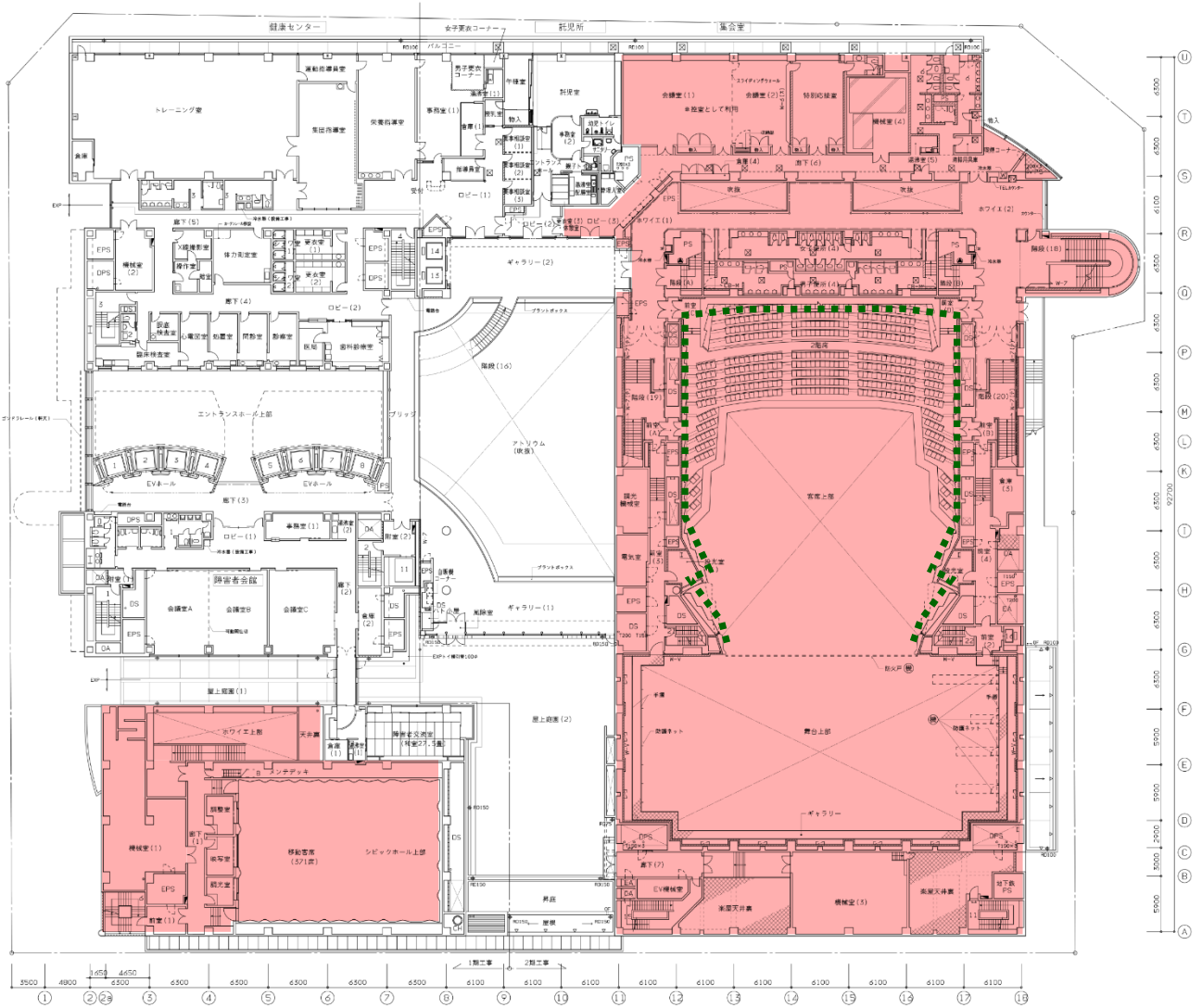
3階平面図
