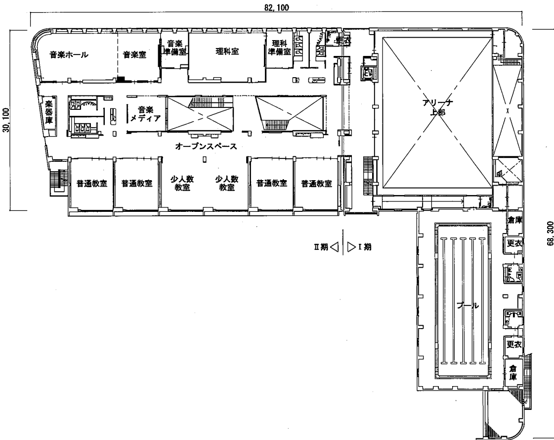
3階平面図
