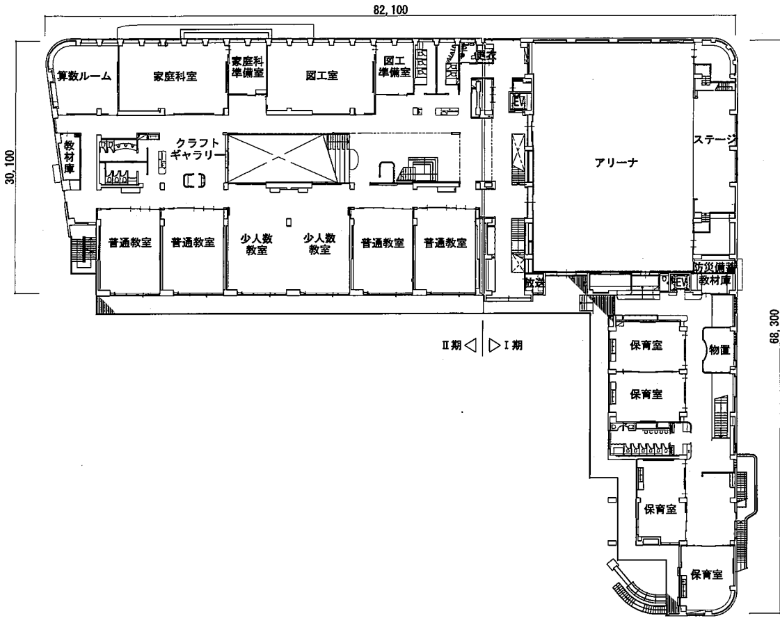
2階平面図
