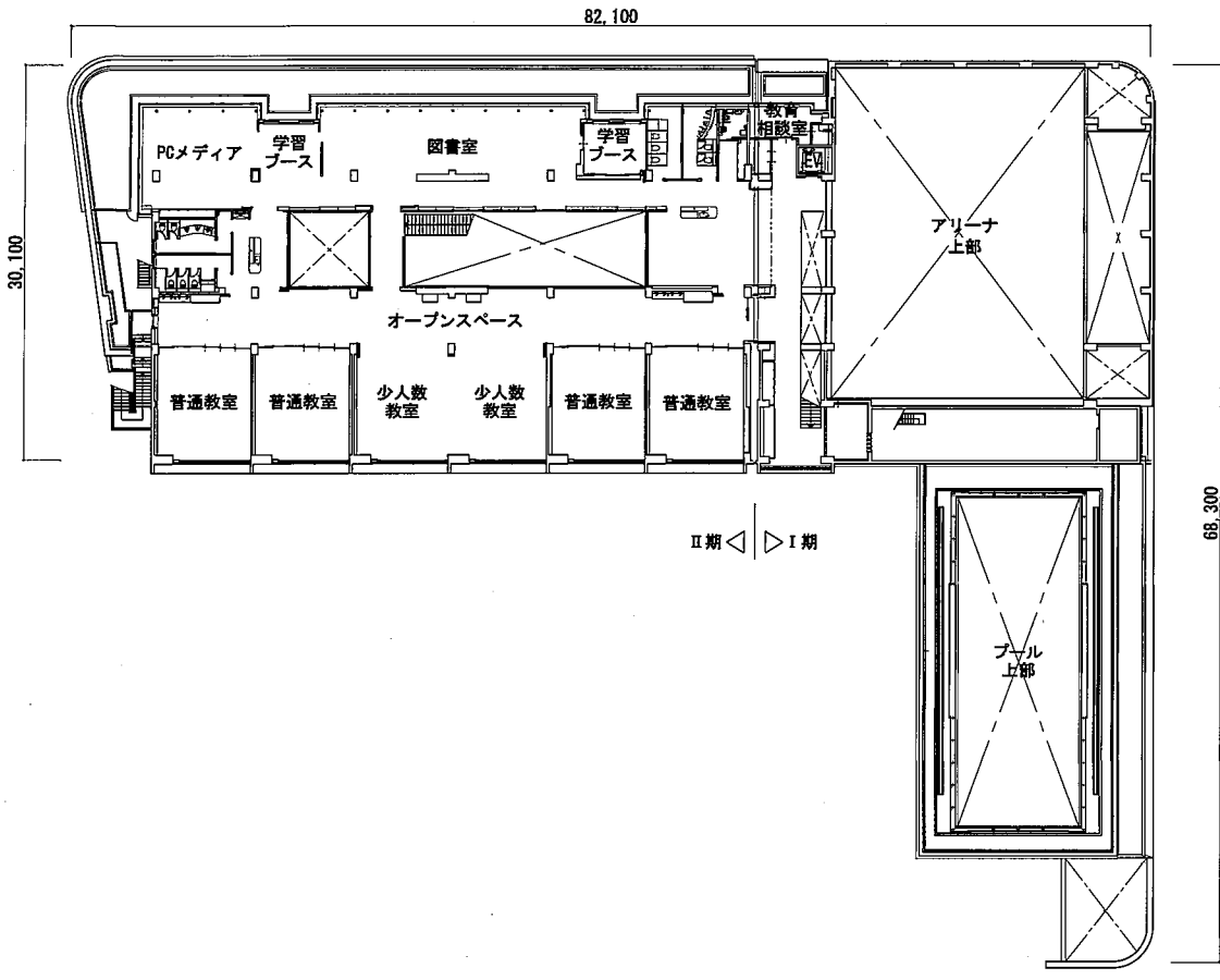
4階平面図
