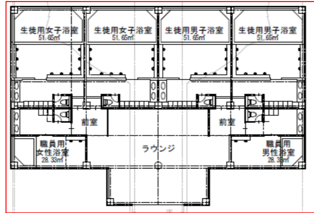
(2階浴室平面図)
