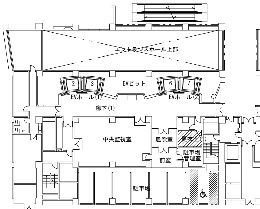
地下1階平面図 (別紙 2 拡大)
