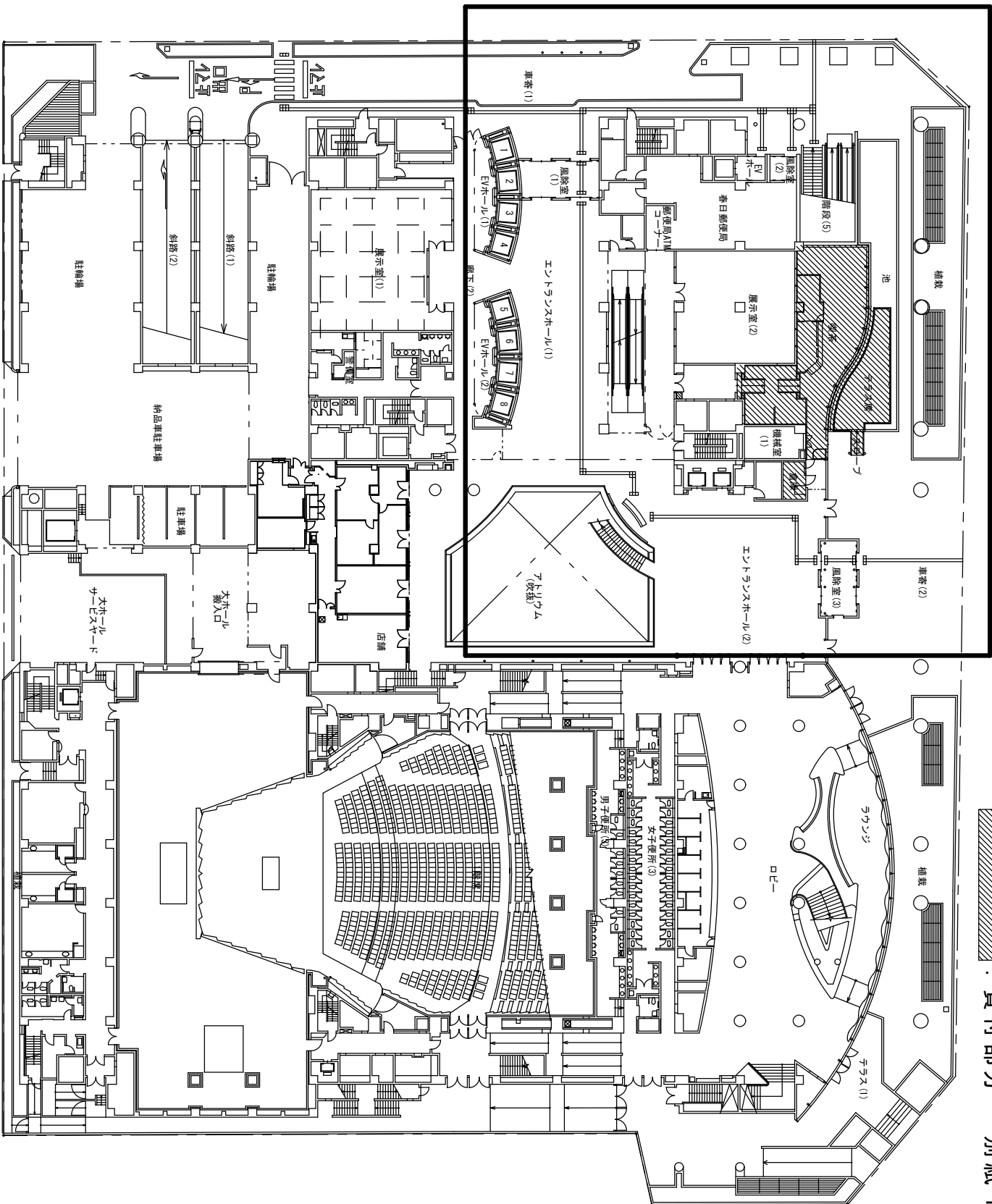
文京シビックセンター1階平面図
