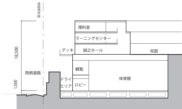
断面図 S=1:500
