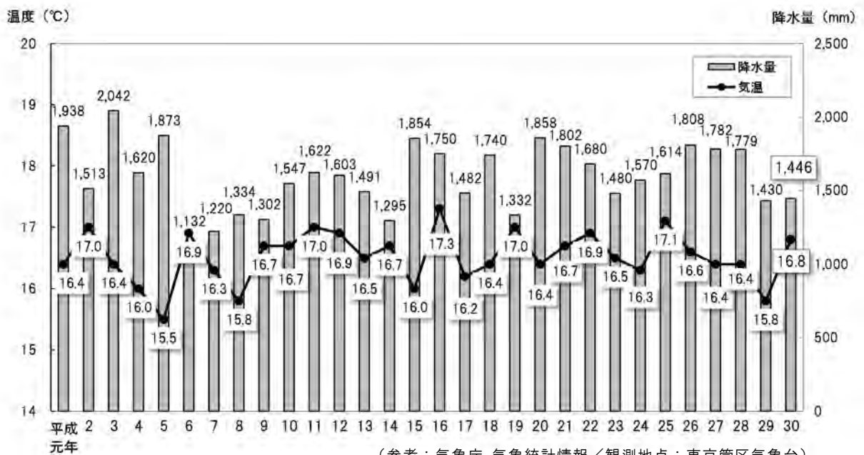
図Ⅱ－３ 文京区付近の過去 30 年の気候推移
