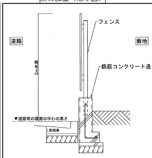
塀の設置（標準図）
