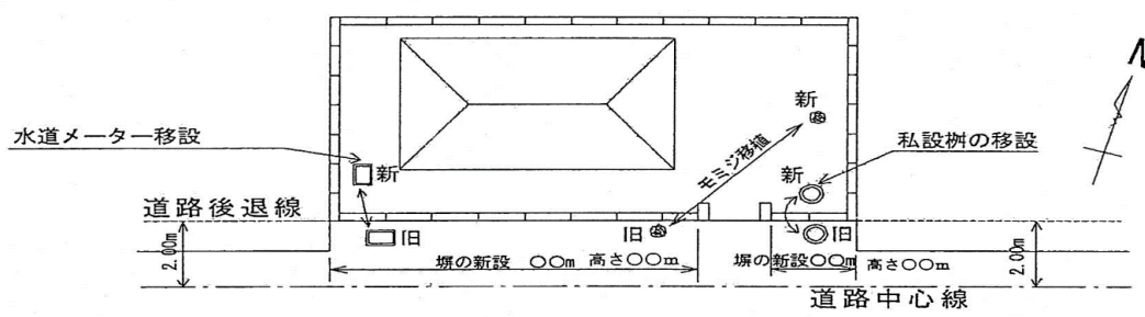
塀の新設・メーターボックス・樹木・私設柵等の移設（工事後）
