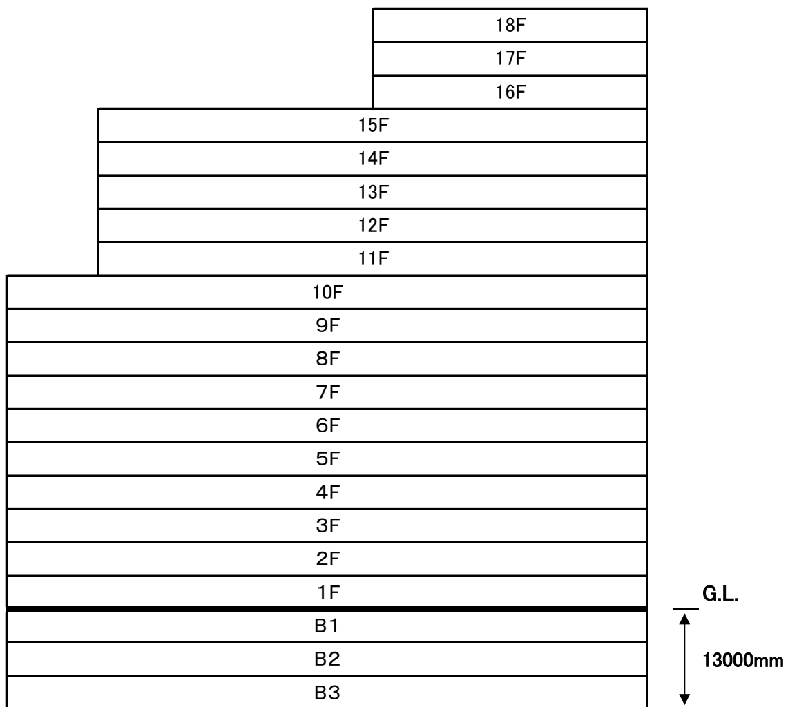
建物立面图（断面）
