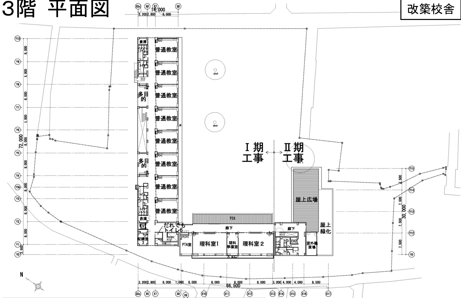
3階平面図
