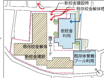
【第2ステップ】 既存校舎解体、新校舎建設(Ⅰ期工事)
