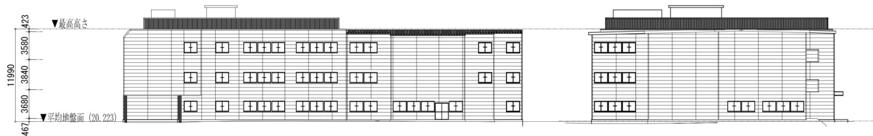
北側立面図
