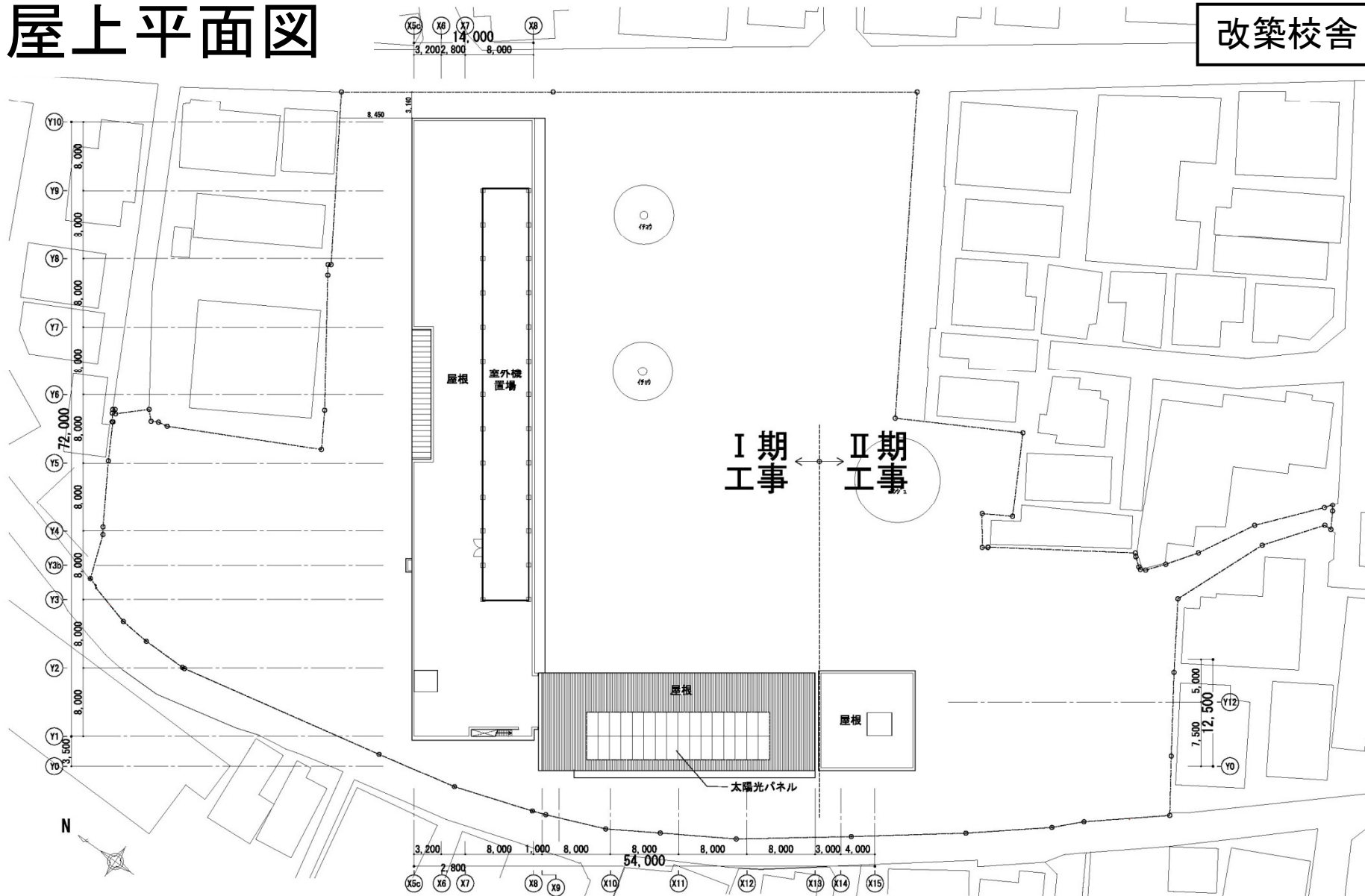
屋上平面図
