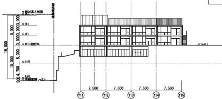
南側立面図-2
