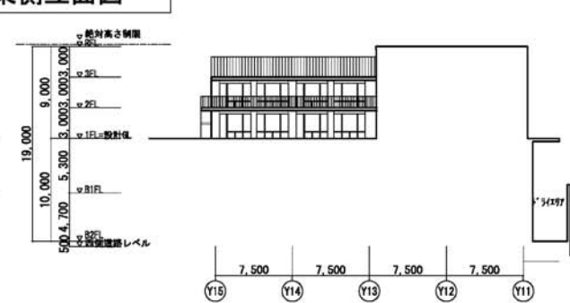
北側立面図-2
