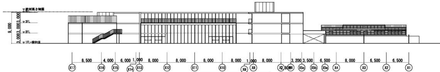
東側立面図
