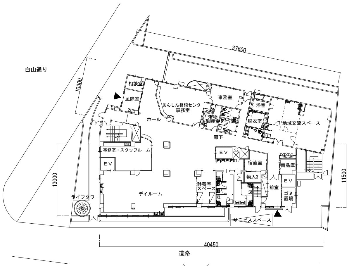
配置図・1階平面図 1/400
