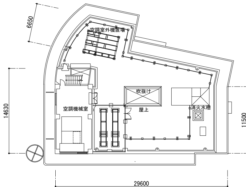
5階平面図 1/400
