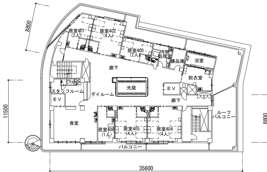
4階平面図 1/400
