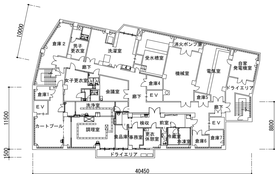
地下1階平面図 1/400
