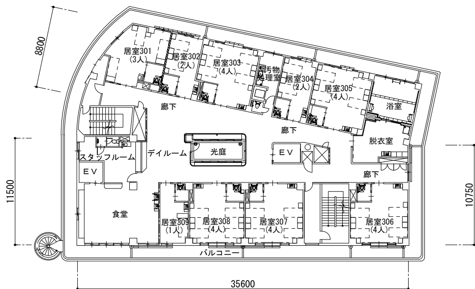
3階平面図 1/400
