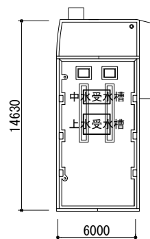
塔屋平面図 1/400
