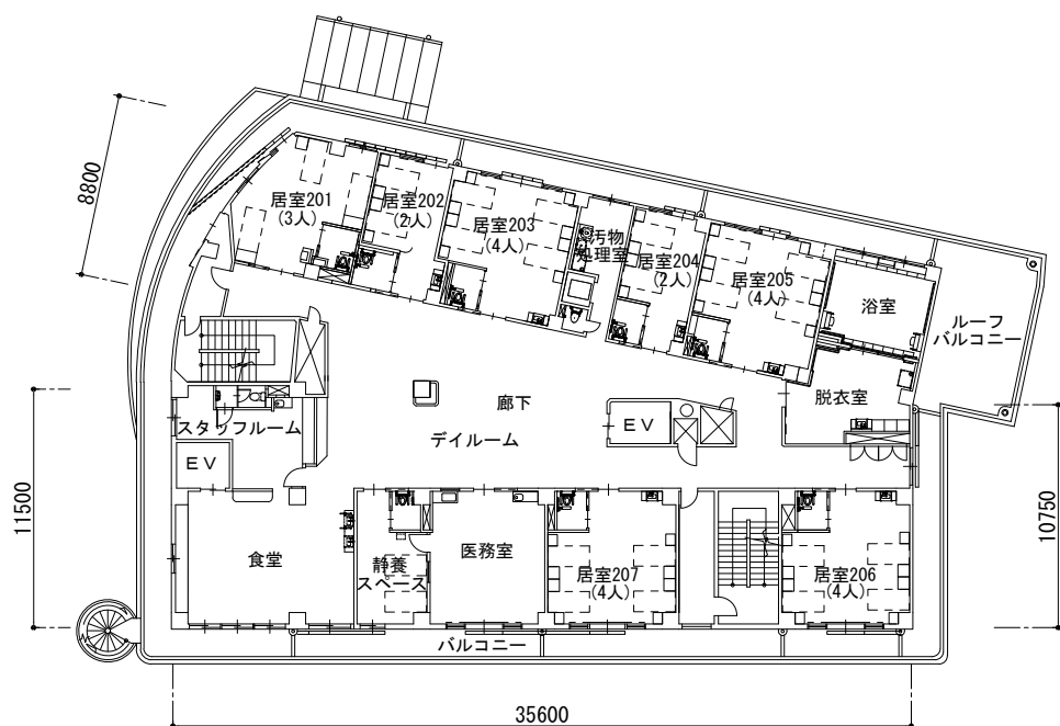
2階平面図 1/400
