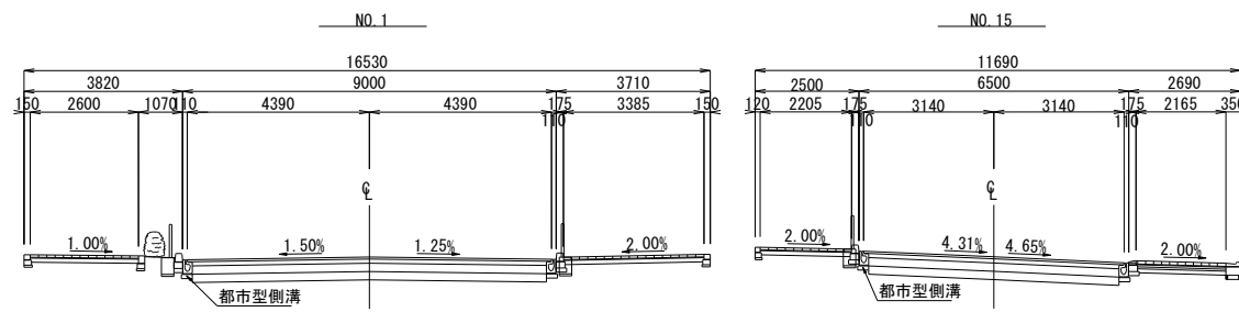
標準横断定規図
