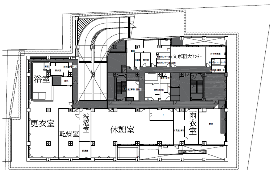
地下1階平面図
