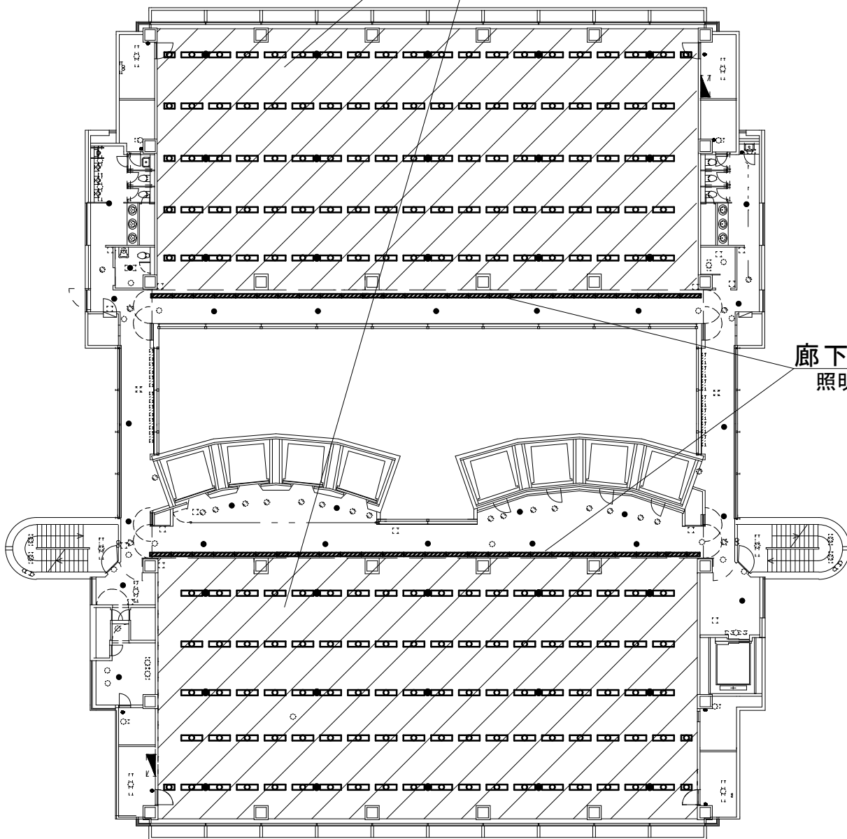
基準階平面図 S=1/300 (例：9階)
