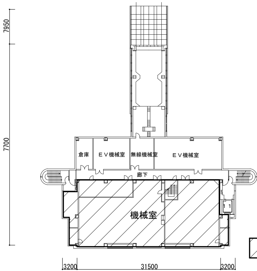
27階平面図 S=1/500
