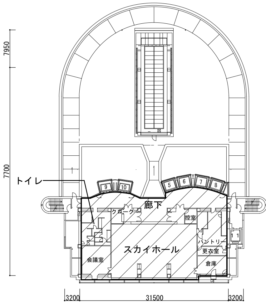
26階平面図 S=1/500
