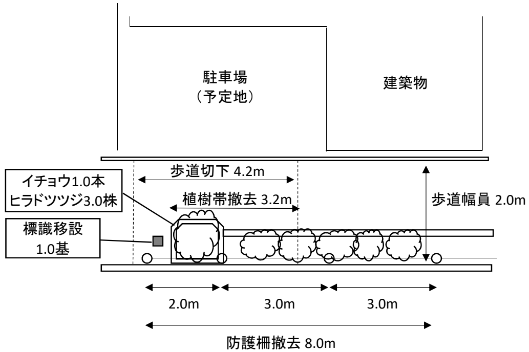
現況平面図
