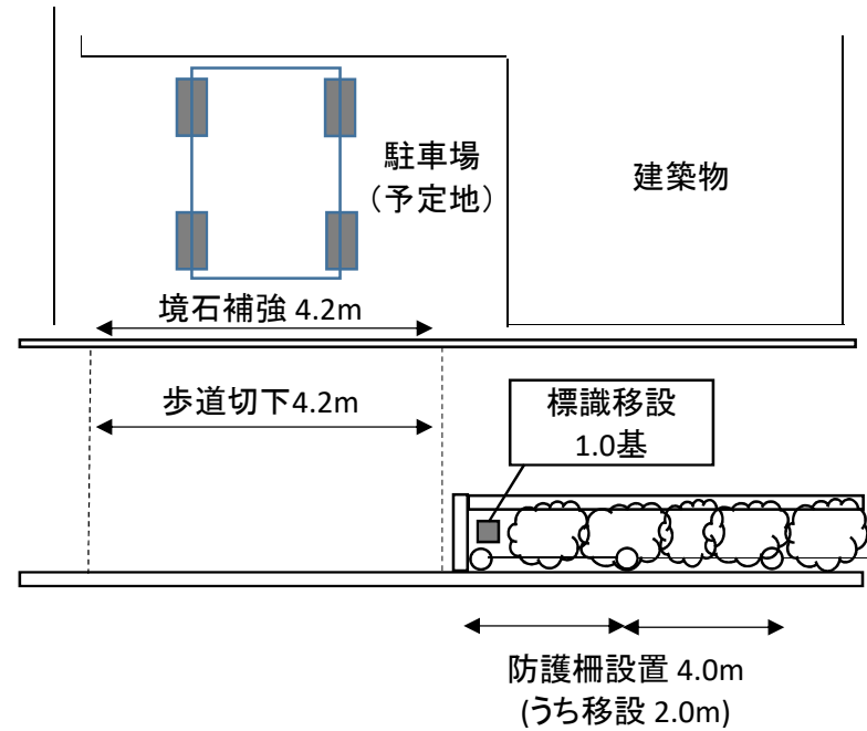
計画平面図
