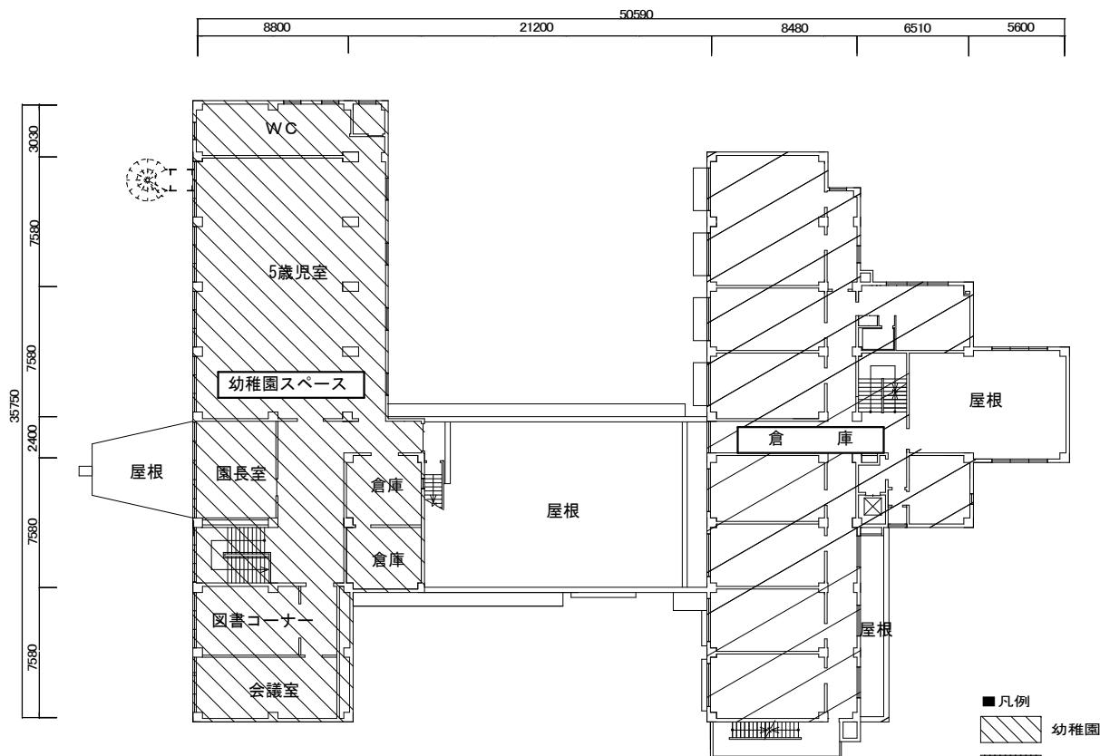
本館 2 階平面図
