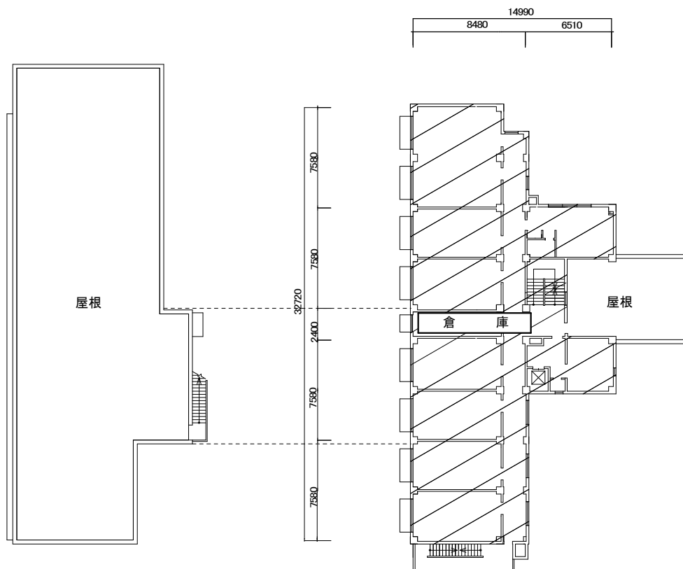
本館 3 階平面図
