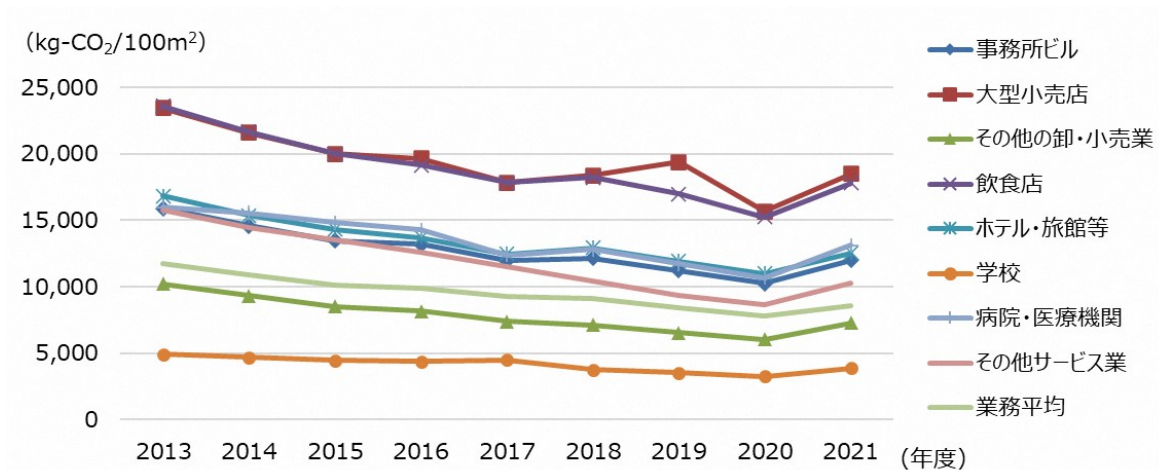
図 36 業種別 床面積 100m 2 当たり二酸化炭素排出量の推移
