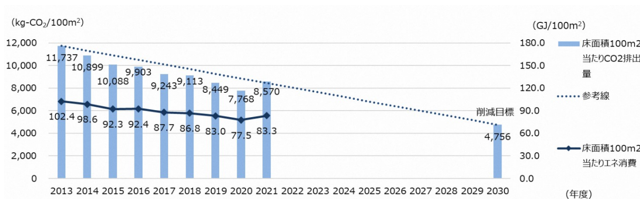
図 35 民生（業務）部門 床面積 100m 2 当たり二酸化炭素排出量とエネルギー消費量の推移
