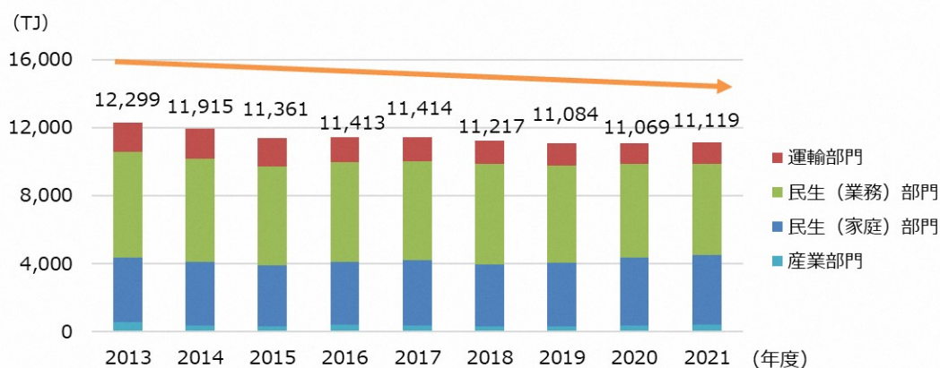
図 28 部門別のエネルギー消費量
